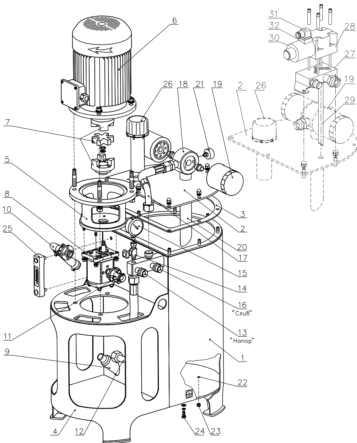
Рис. 5. Установка насосная.
