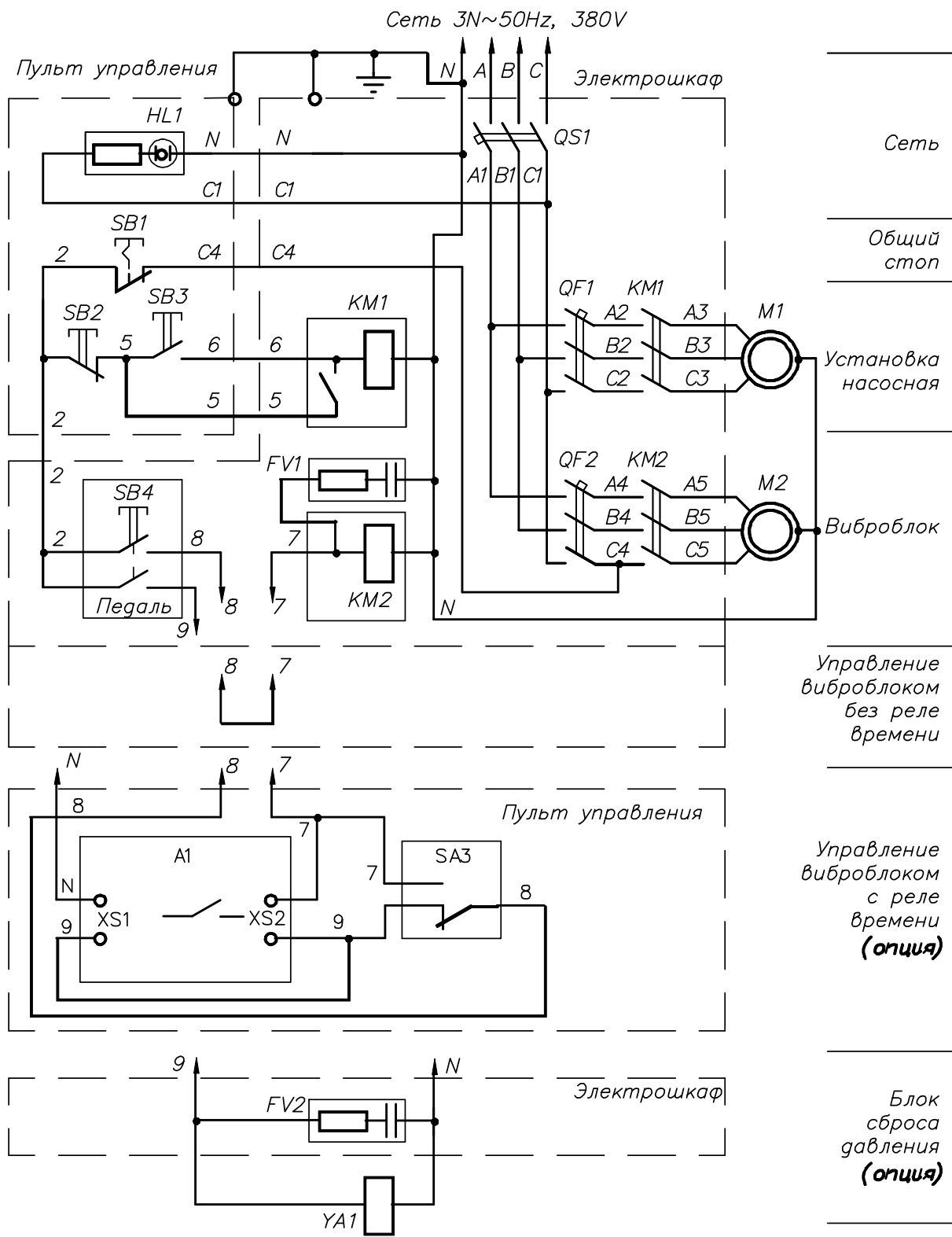
Рис. 8 .Схема электрическая принципиальная.
