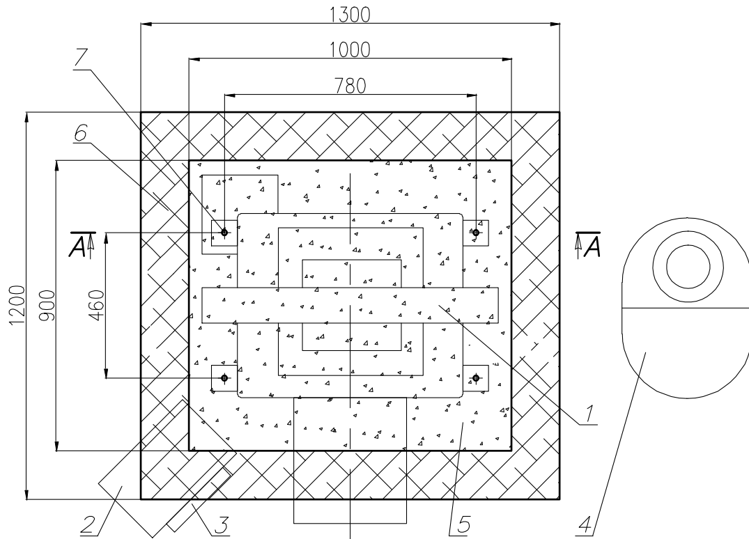
Рис. 10. План фундамента вибропресса.
