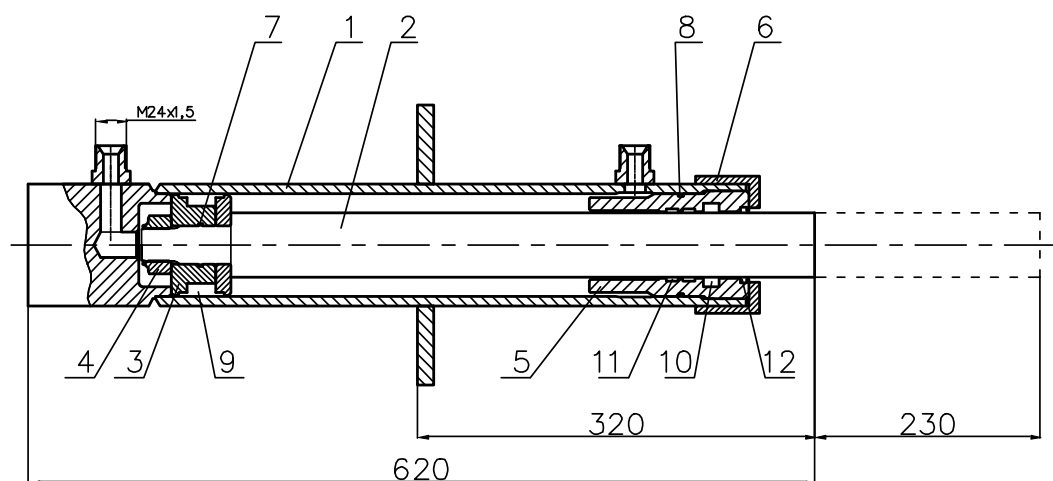
Рис. 7. Гидроцилиндры.
