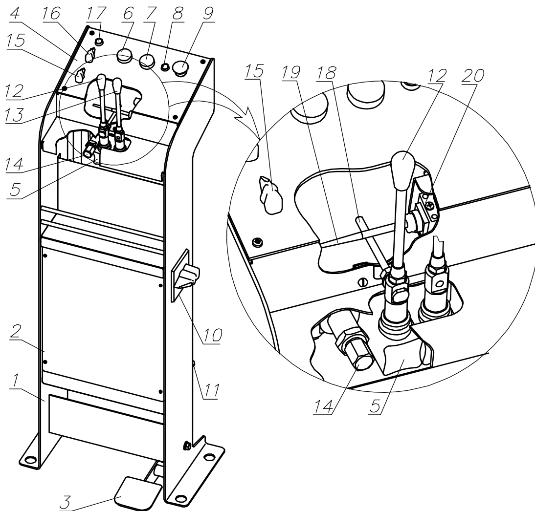
Рис. 3 Пульт управления.
