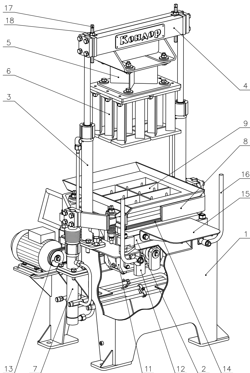
Рис.2. Вибропресс.
