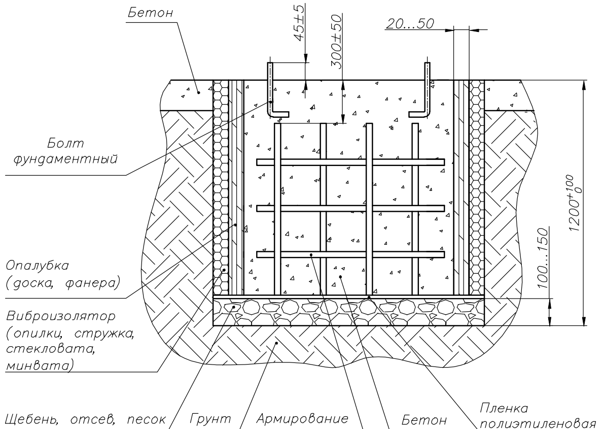
Рис. 11. Сечение фундамента по АА.
